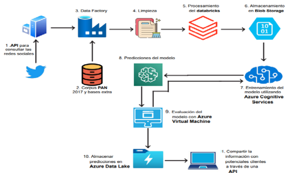
Figura 3 Arquitectura del proyecto.
