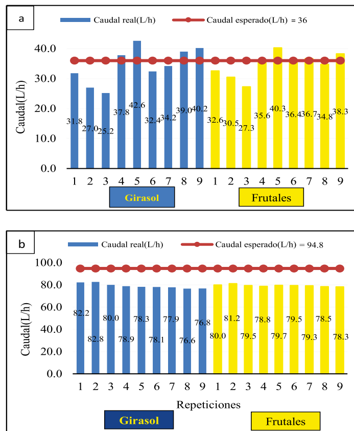
Figura 12 Caudal promedio del FBA(a), FLAI(b)
